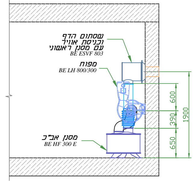
חֶתֶךְ 1-1
