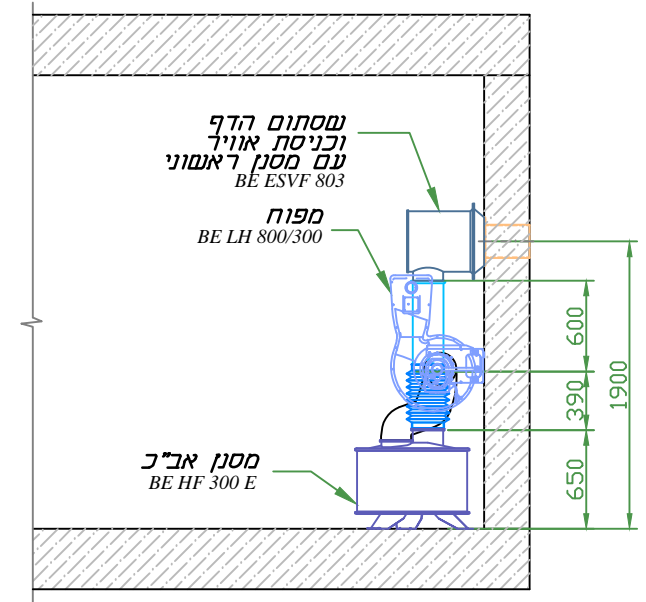
חתך 1-1
