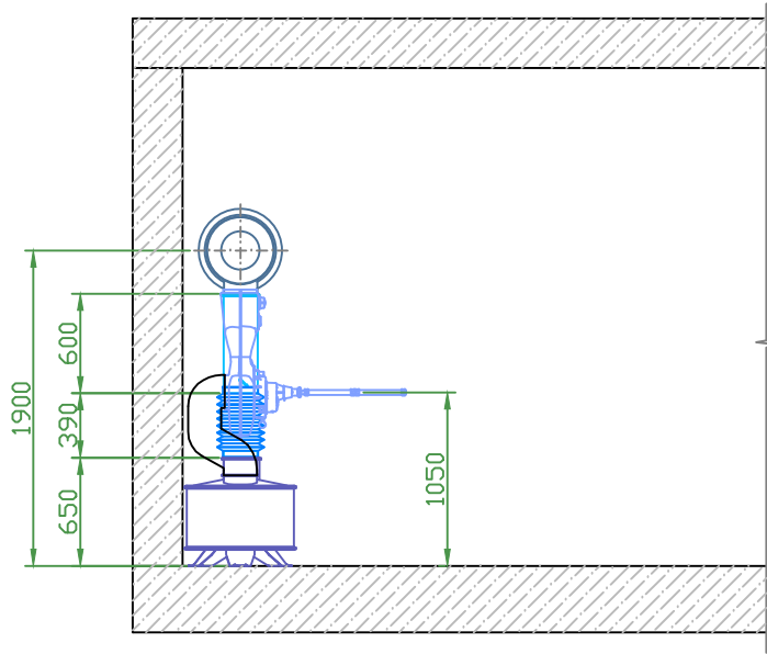
חתך 1-1
