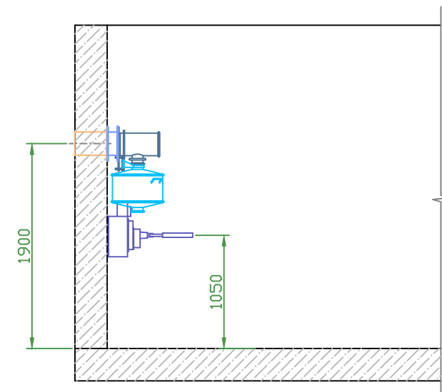
חתך 1-1
