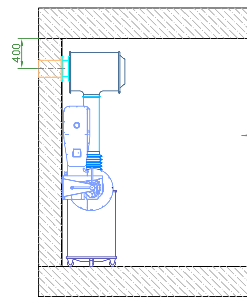
חתך 1-1
