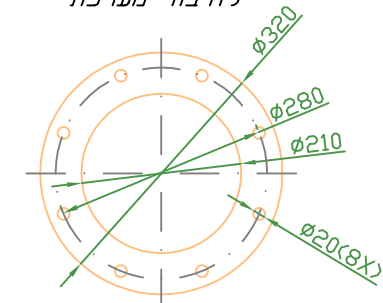
חתך 2-2 קנ"מ 1:10
