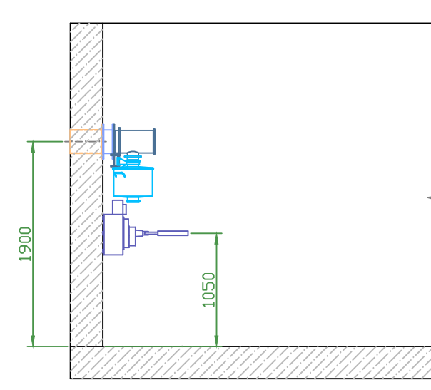
חתך 1-1
